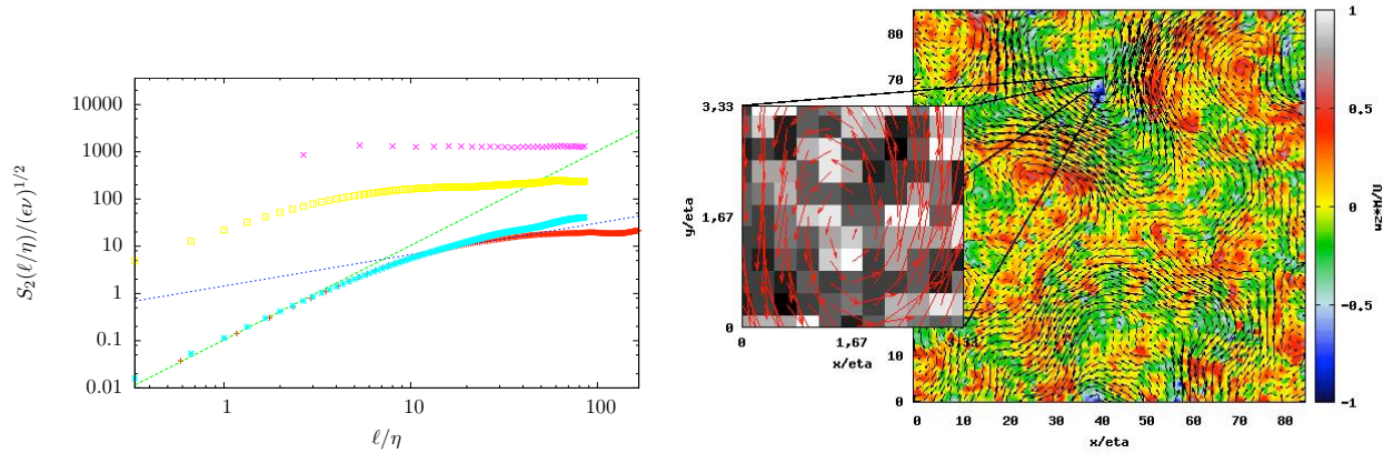
FIGURE 2 – Turbulence de grille. A gauche, Comparaisons de fonctions de structure d’ordre 2. Rouge, mesures fil-chaud ; Turquoise, méthode proposée ; Jaune, approche de [7] ; Fuchsia ; corrélation ; Tiret vert, \sim \ell^2 ; Tiret bleu, \sim \ell^{(2/3)} . A droite, champs de vecteurs avec vorticité et images de particules estimés avec la méthode proposée.
