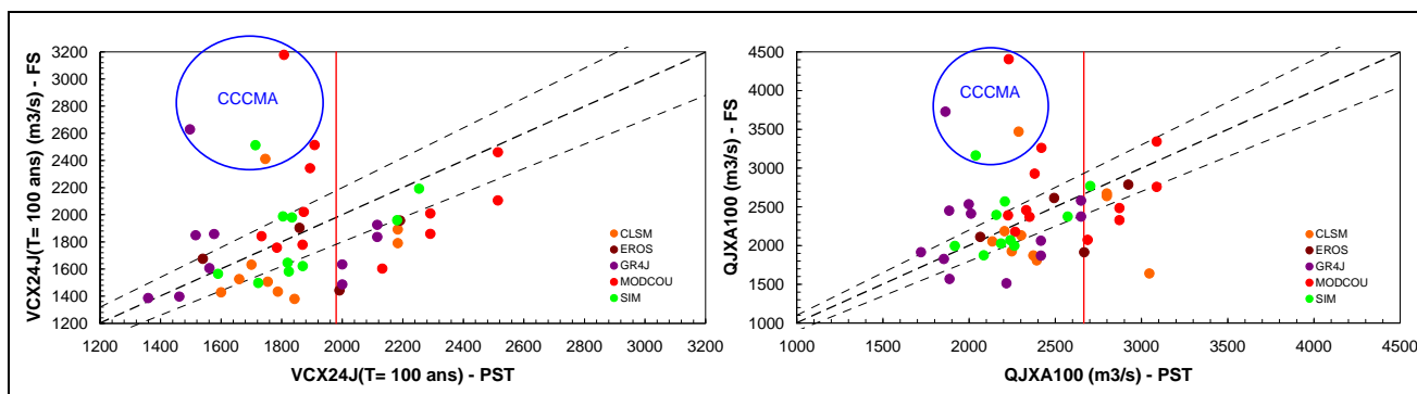
Figure 5 - Evolution des quantiles centennaux du débit à Paris entre le climat présent (PST) et la fin du siècle (FS) : débits moyens sur 24 jours VCX24J(T=100 \text{ ans}) et débits journaliers QJXA100 . Un point par scénario hydrologique. La droite en tireté est la première bissectrice et celles en pointillé définissent les enveloppes à \pm 10\% des valeurs PST. La droite verticale rouge donne les quantiles centennaux déduits des observations de débit [14].
