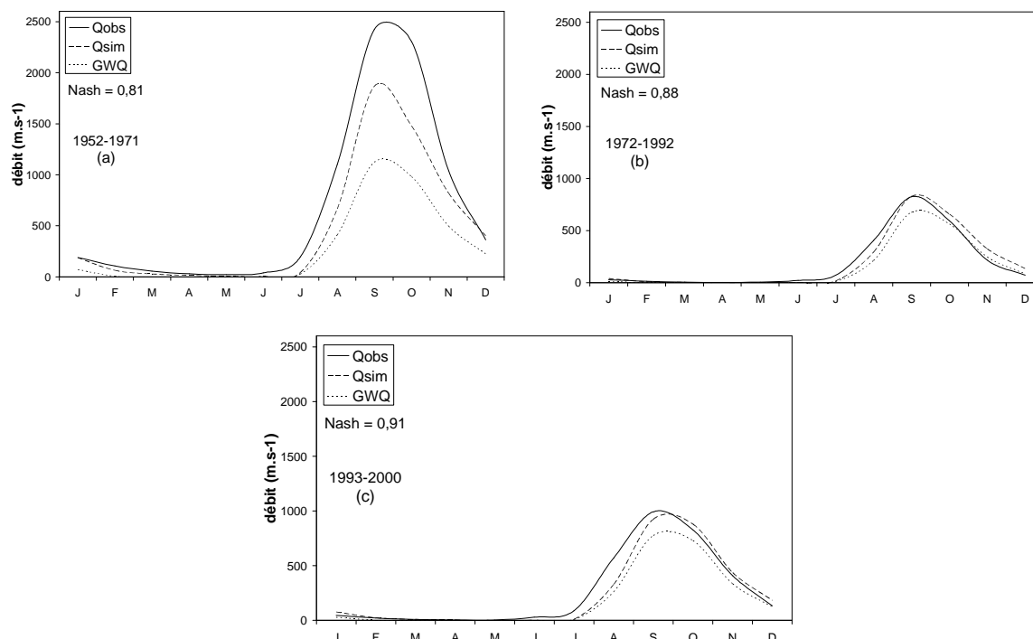
Fig. 3 Moyennes mensuelles des débits mesurés Q_{\text{obs}} et simulés Q_{\text{sim}} , et des débits de base simulés GWQ (générés par les nappes souterraines) à Douna : (a) 1952-1971; (b) 1972-1992 ; (c) 1993-2000.
