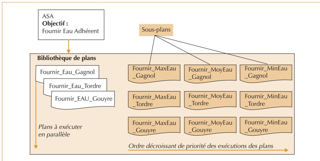
Figure 7 – Plans exécutés en parallèle et en séquentielle.
